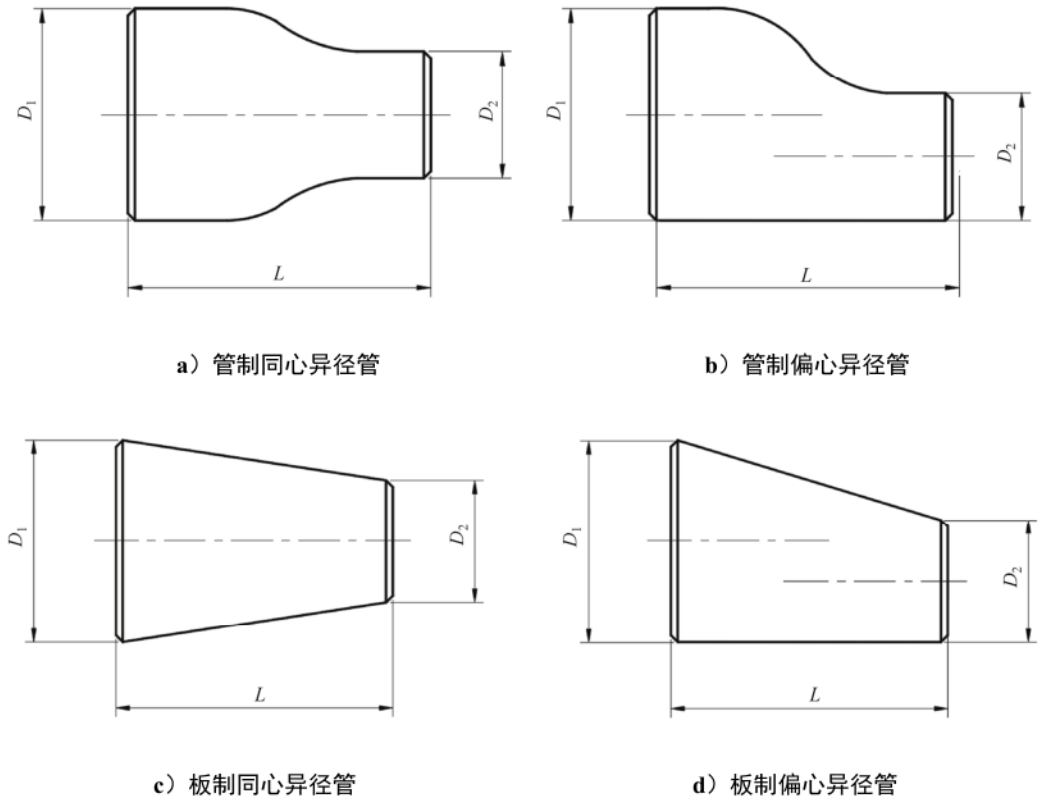
图 4.1.4 异径管外形
