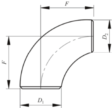
图 4.1.10 异径弯头外形
