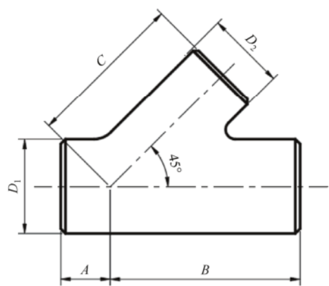
图 4.1.8 45° 异径 Y 型无缝三通外形
