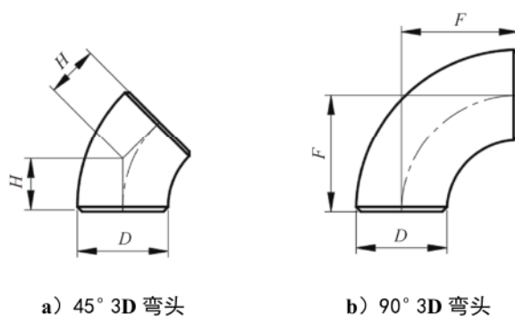
图 4.1.2 45° 3D 弯头和 90° 3D 弯头外形
