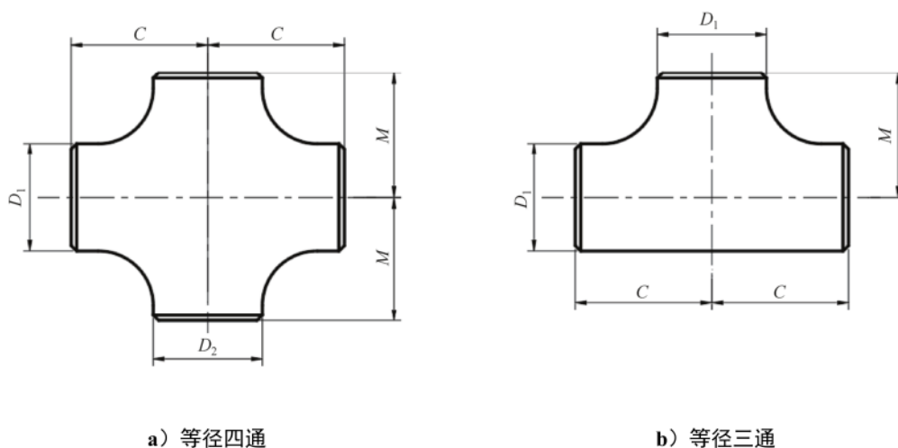
图 4.1.5 等径三通和等径四通外形
