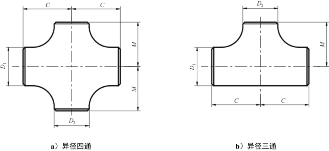
图 4.1.6 异径三通和异径四通外形
