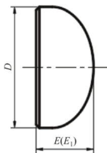
图 4.1.9 管帽外形
