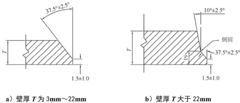
图 6.1.4 坡口尺寸和形状
