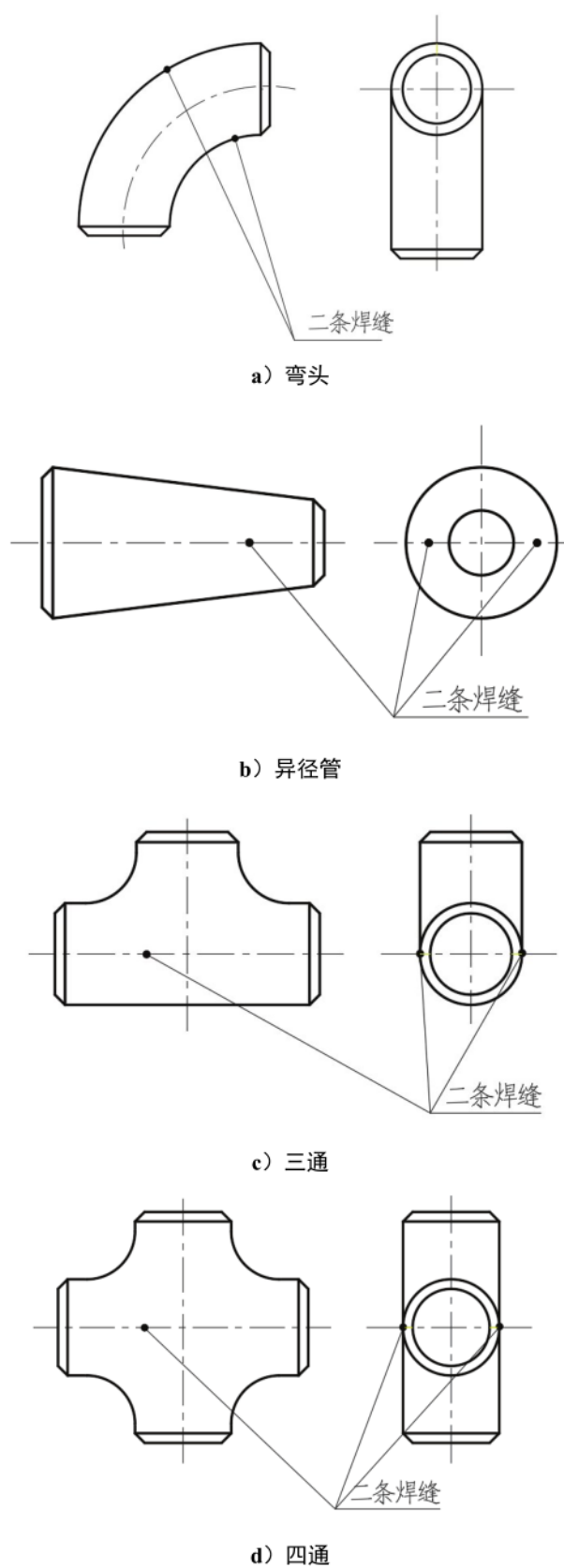
图 6.1.6 管件上焊缝的位置
