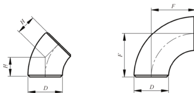
a) 45° 弯头
