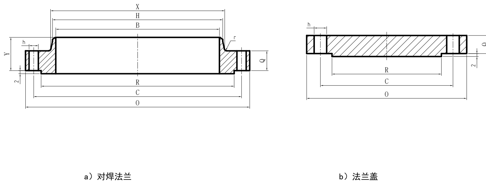
图 4.5.3 Class300 B 系列法兰结构型式
