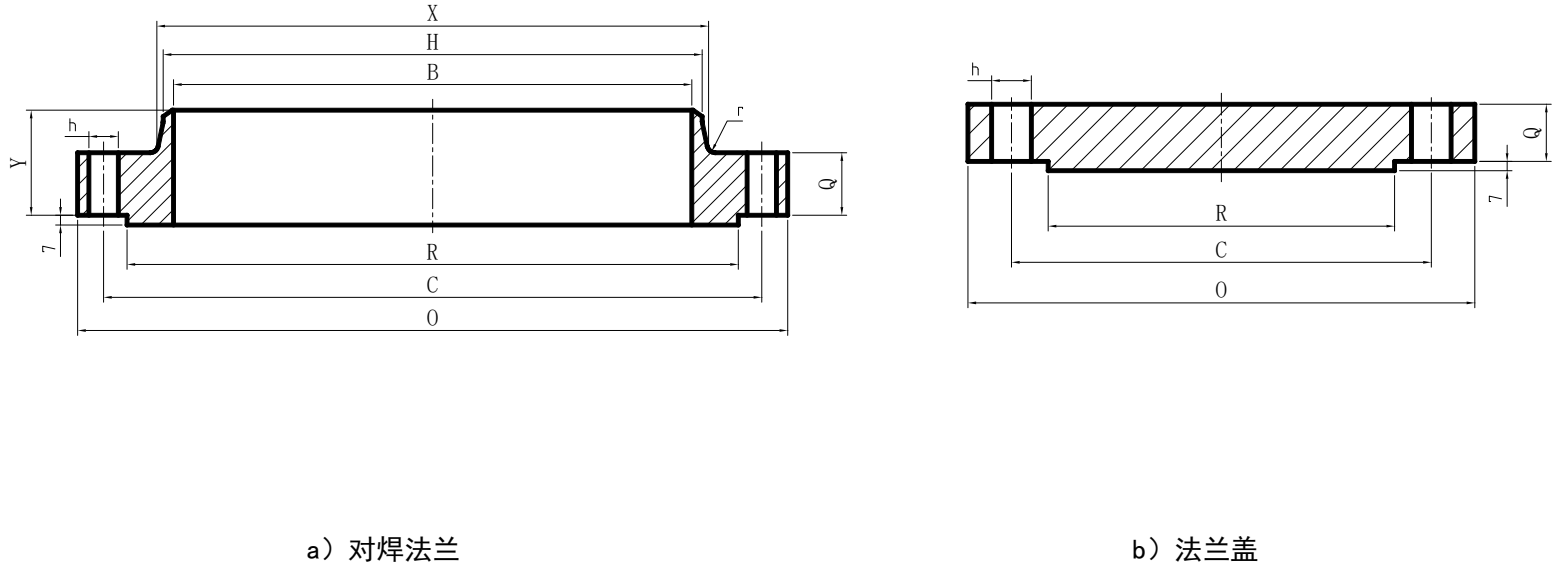
图 4.5.5 Class900 B 系列法兰结构型式
