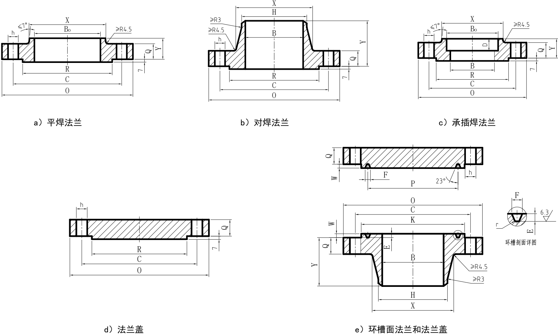
图 4.1.4 Class600 法兰结构型式
