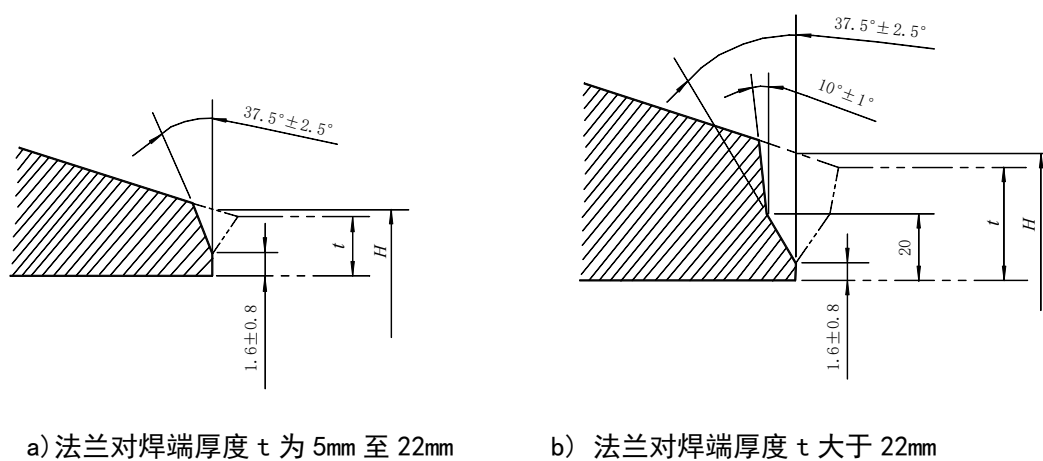
图 4.7.2 公称直径 DN > 600\text{mm} 对焊法兰焊接端坡口
