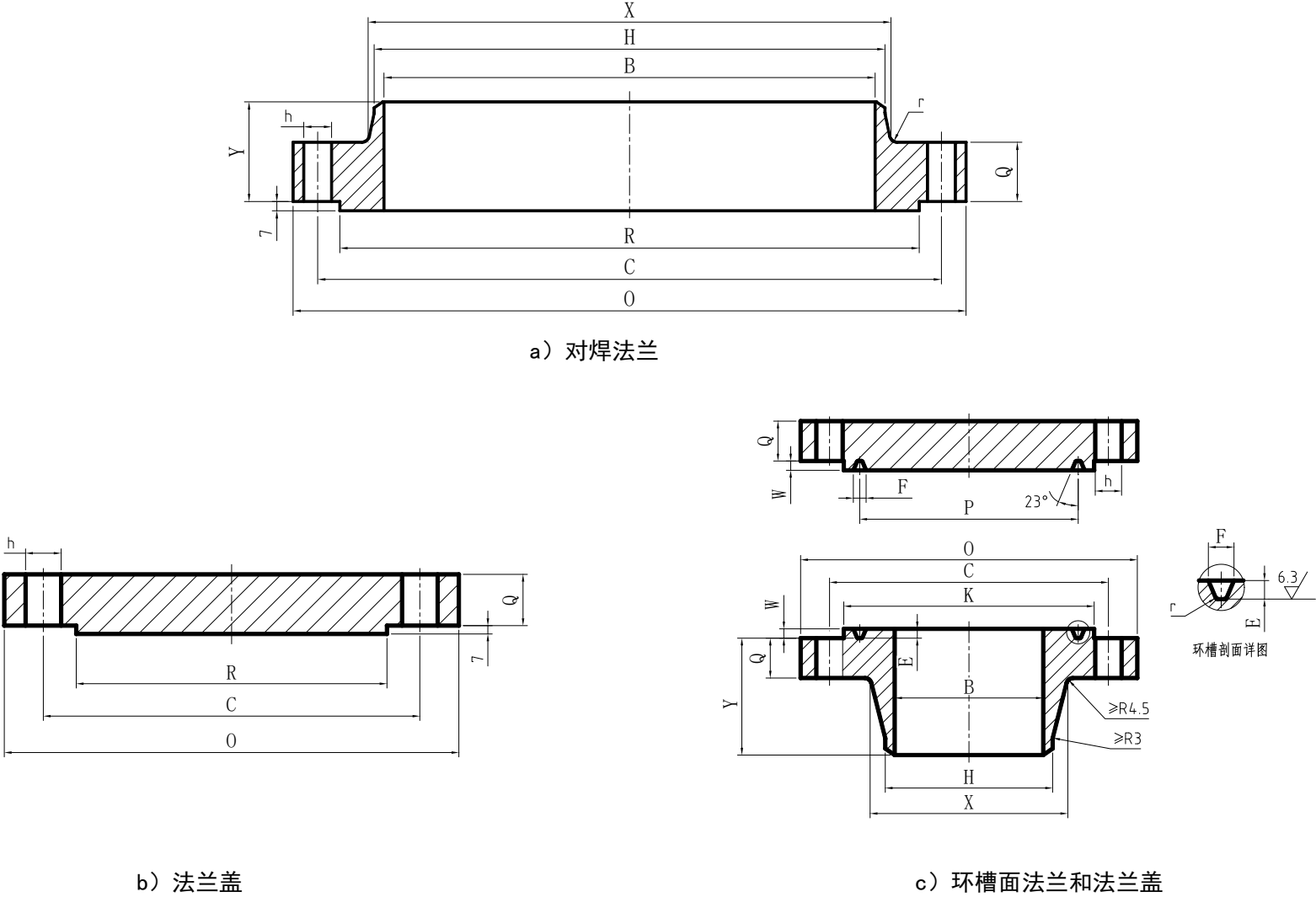
图 4.4.3 Class600 A 系列法兰结构型式
