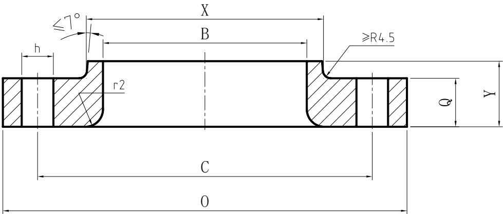
图 4.2.4 PN110 (Class600) 松套法兰结构型式
