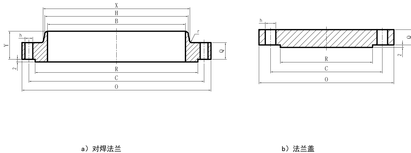
图 4.5.2 Class150 B 系列法兰结构型式
