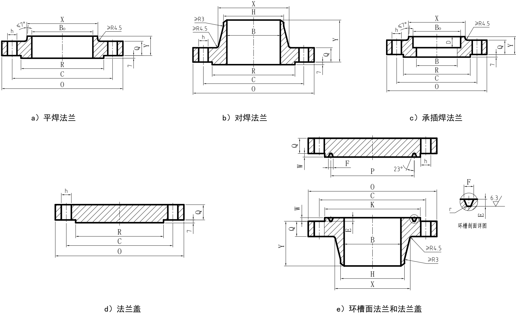
图 4.1.5 Class900 法兰结构型式
