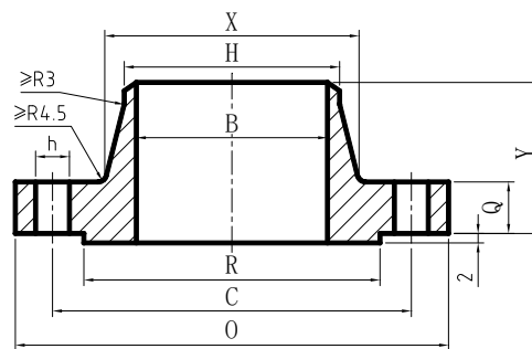
b) 对焊法兰
