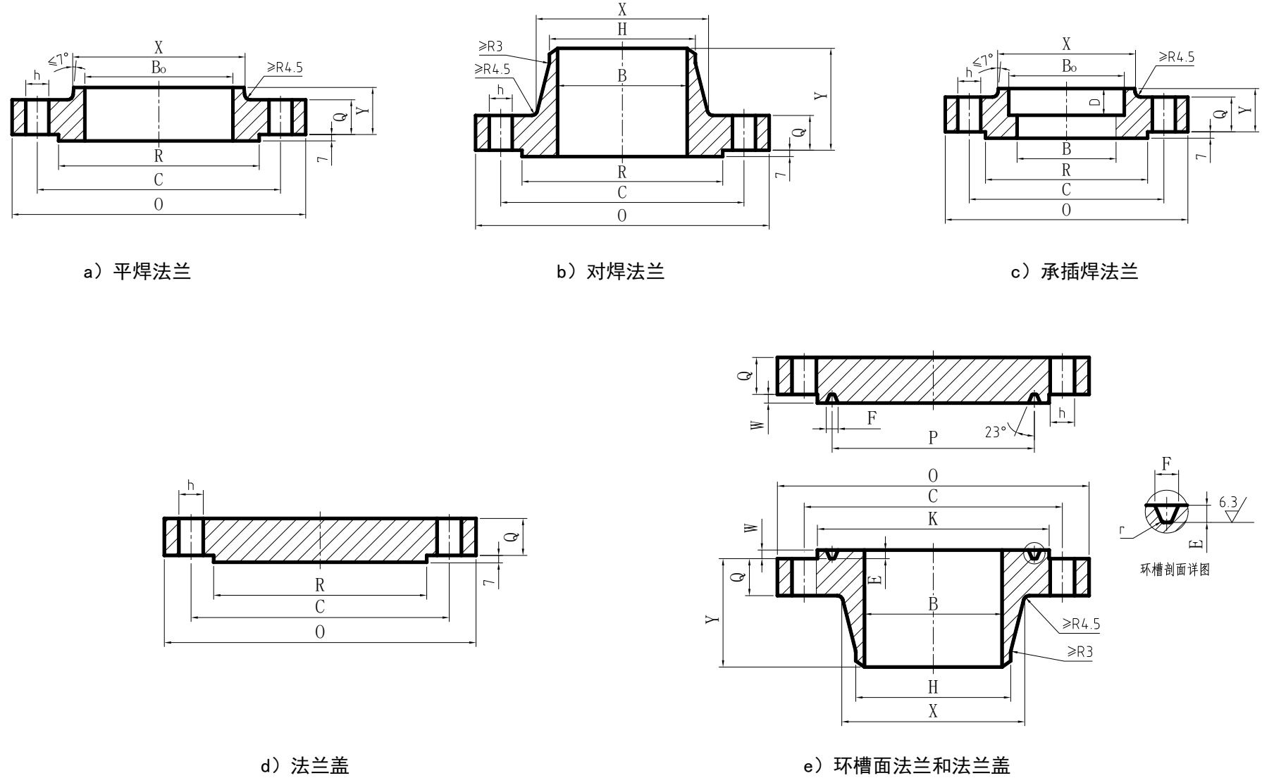
图 4.1.6 Class1500 法兰结构型式
