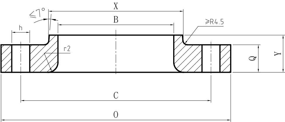
图 4.2.2 Class300 松套法兰结构型式
