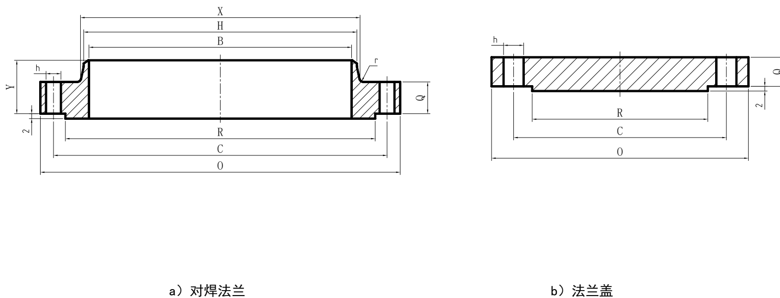
图 4.5.1 Class75 B 系列法兰结构型式
