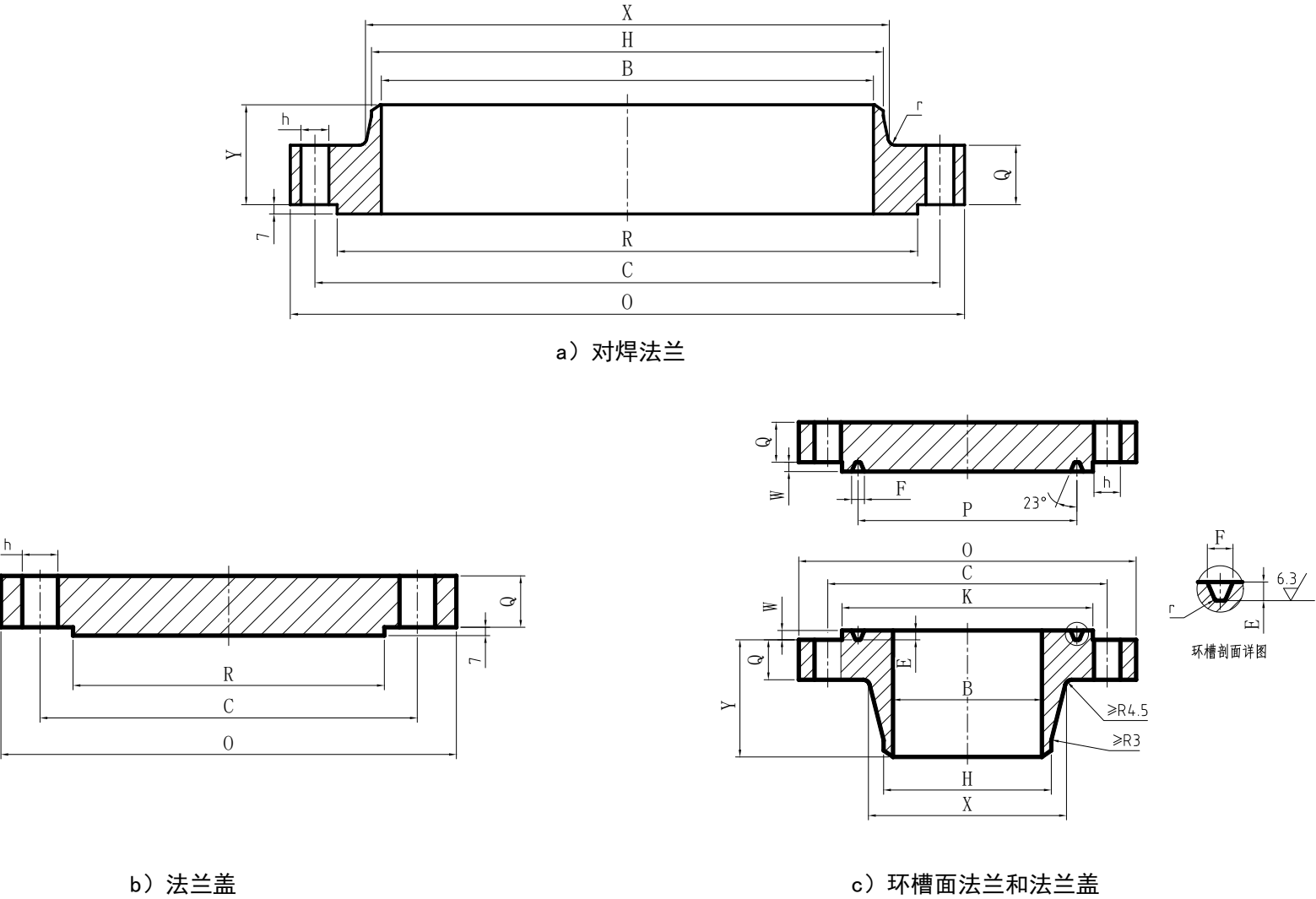
图 4.4.4 Class900 A 系列法兰结构型式
