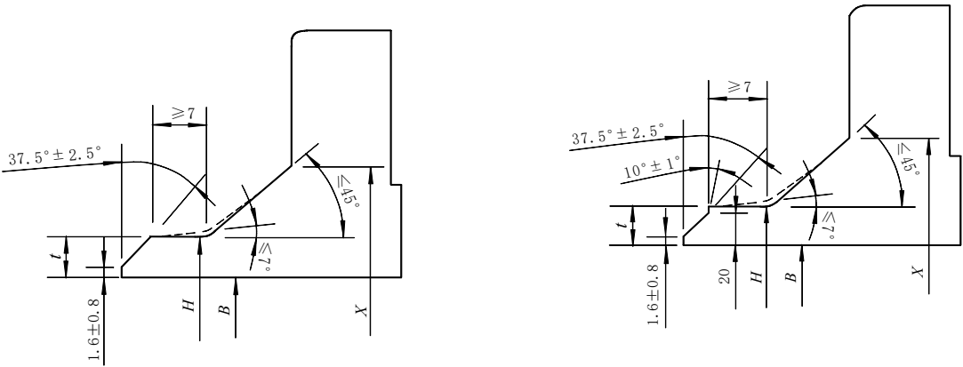
a) 法兰对焊端厚度 t 为 5mm 至 22mm b) 法兰对焊端厚度 t 大于 22mm
