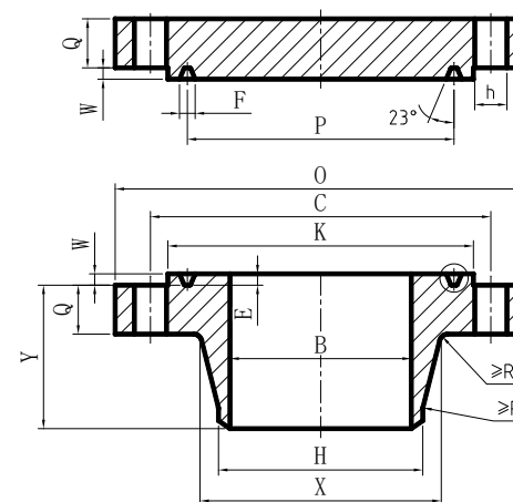
f) 环槽面法兰和法兰盖
