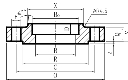
c) 承插焊法兰
