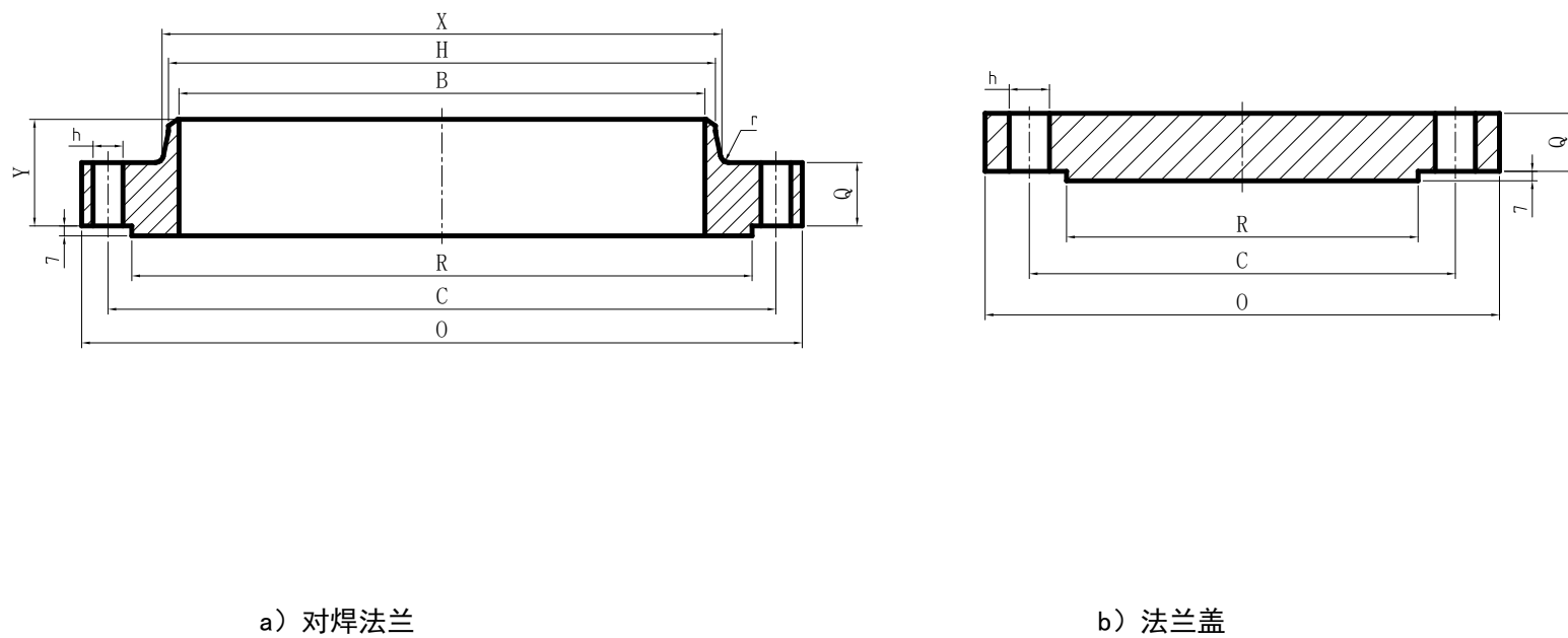
图 4.5.4 Class600 B 系列法兰结构型式
